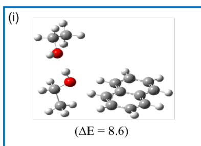
(c) C 10 H 8 •+ (EtOH) 3
